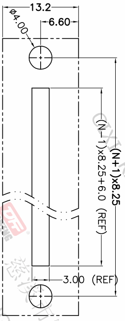
P.C.B.LAYOUT
