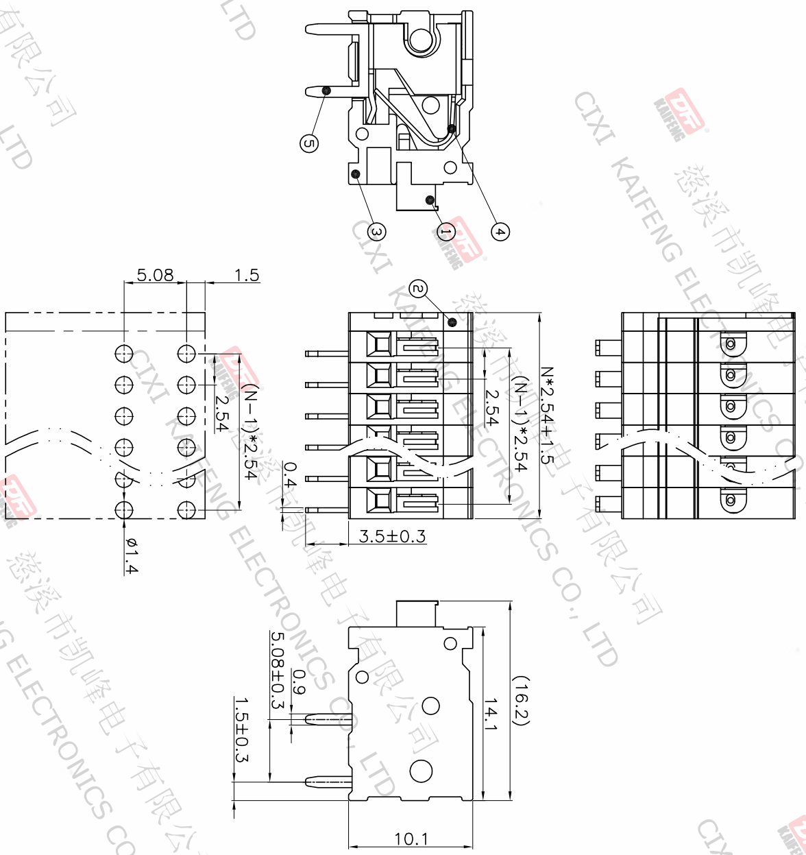
P.C.B.LAYOUT
