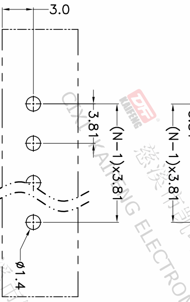
P.C.B. LAYOUT
