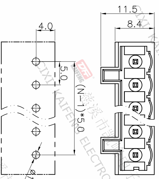
P.C.B.LAYOUT
